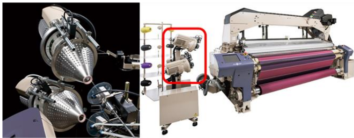
よこ入れ装置：エアジェットルームの横に設置し、送り込む「よこ糸」の長さを測ります。
